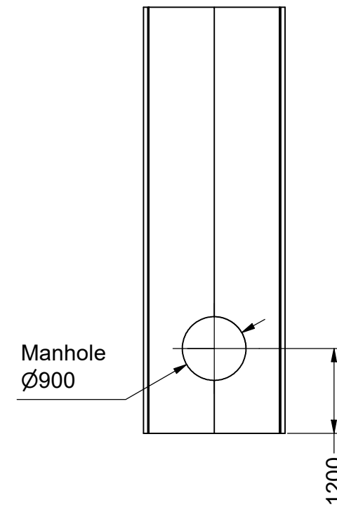
C-C ( 1 : 100 )
