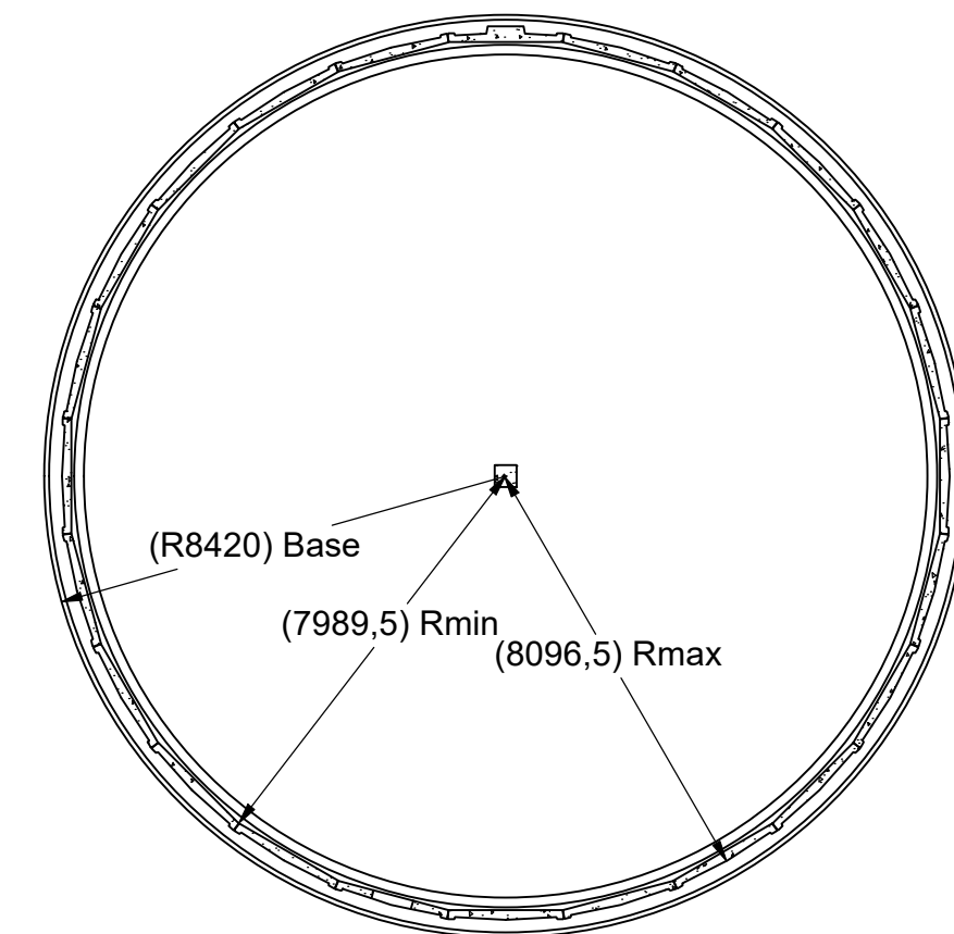
D-D ( 1 : 150 )
