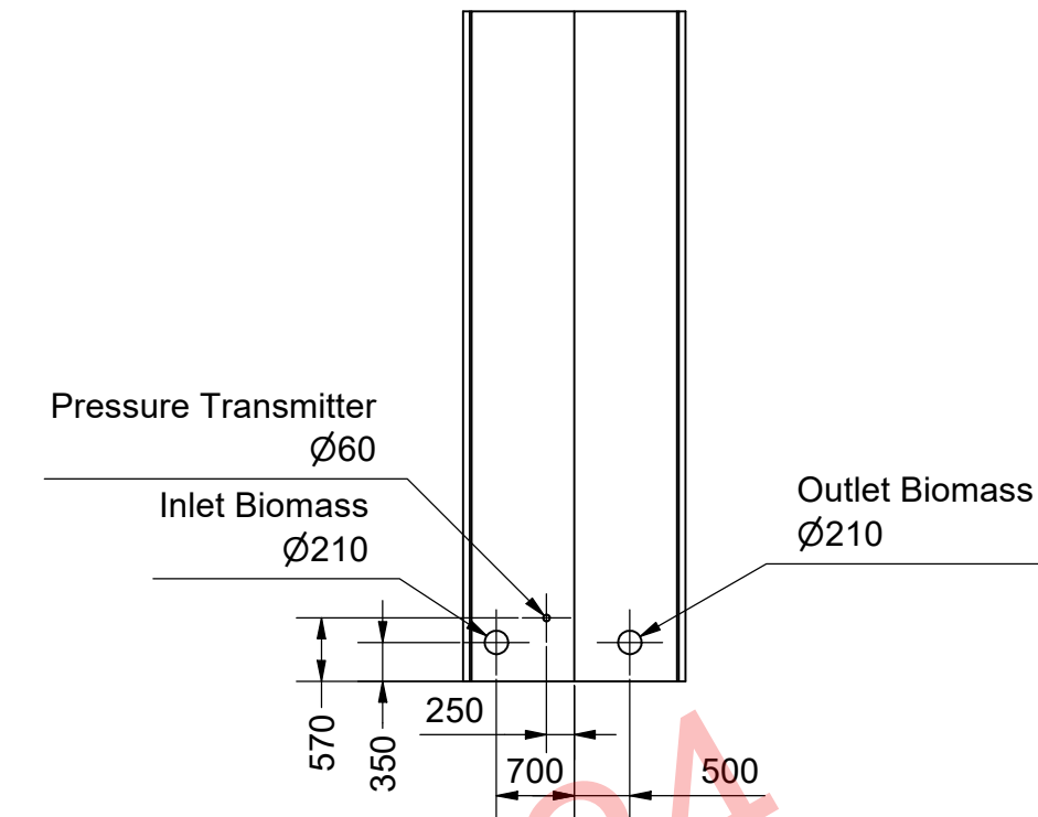
D-D ( 1 : 150 )
